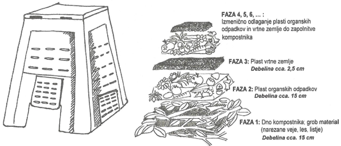
Slika 5 : Proces kompostiranja
